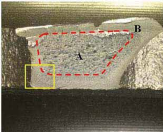
Riduttore dell'elica di un P92: particolare analisi superficie di frattura con presenza di dimples nella zona "A" e di una crinatura perpendicolare alla superficie di rottura nella zona "B". La foto a destra è un ingrandimento della zona evidenziata in giallo.
