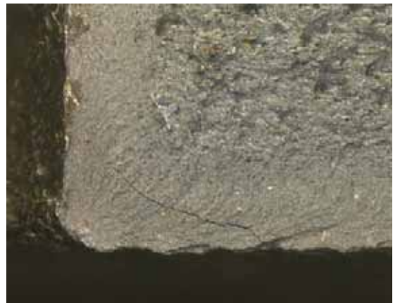
Riduttore dell'elica di un P92: particolare analisi superficie di frattura con presenza di dimples nella zona "A" e di una crinatura perpendicolare alla superficie di rottura nella zona "B". La foto a destra è un ingrandimento della zona evidenziata in giallo.
