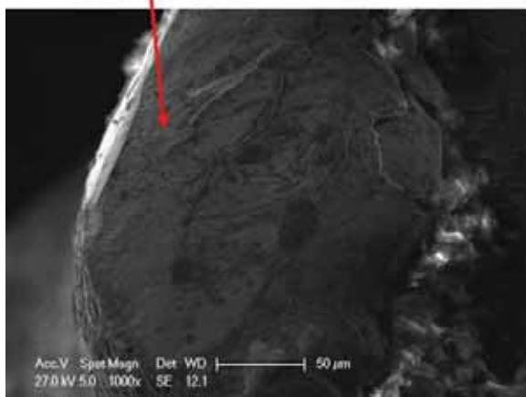
Motore Ivchenko Progress D18-T: analisi superficie di frattura tramite microscopio elettronico.
